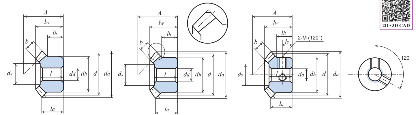
Fig. 1 (Tip chamfering)
