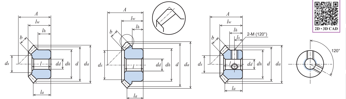
Fig. 1 (Tip chamfering)
