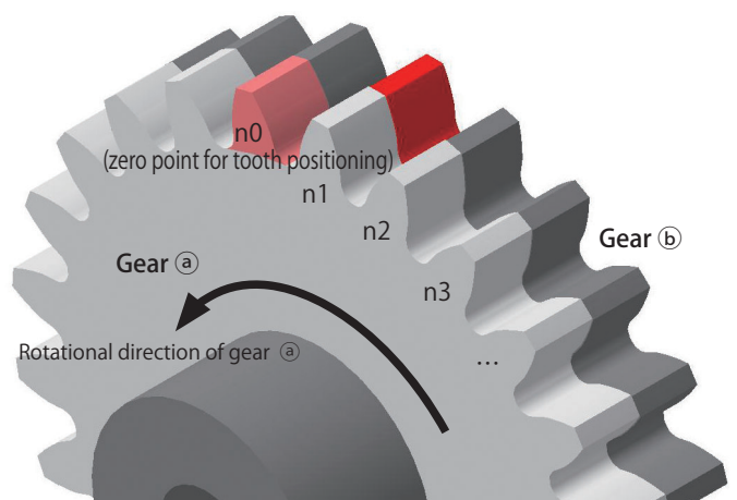
Fig. 3 Pitch shift
