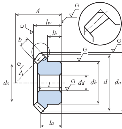
Fig. 1 (Tip chamfering)
