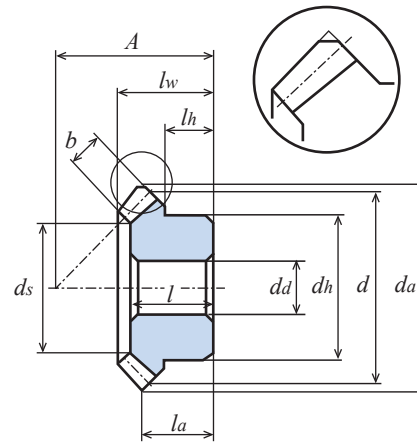
Fig. 1 (Tip chamfering)
