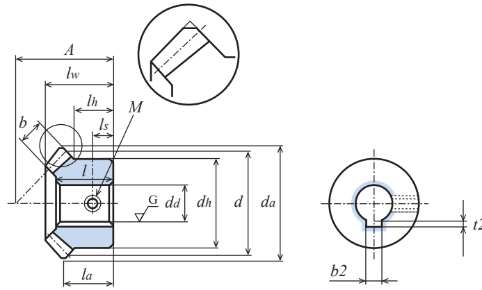
Fig. 1 (Tip chamfering)
