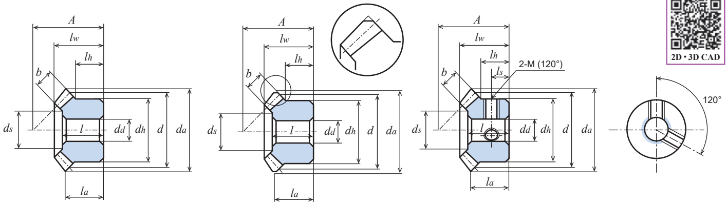
Fig. 1 (Tip chamfering)
