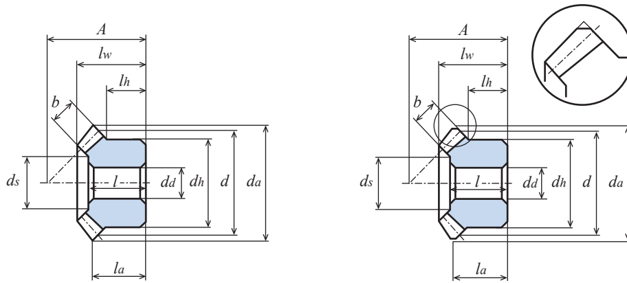
Fig. 1 (Tip chamfering)
