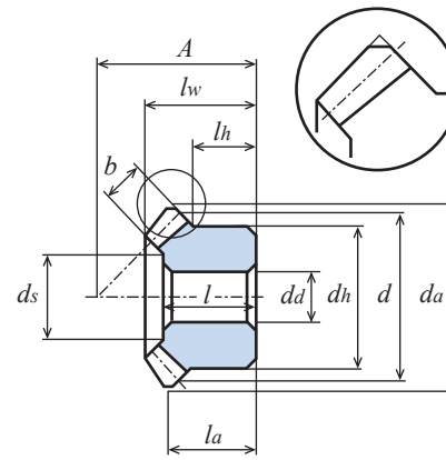
Fig. 1 (Tip chamfering)
