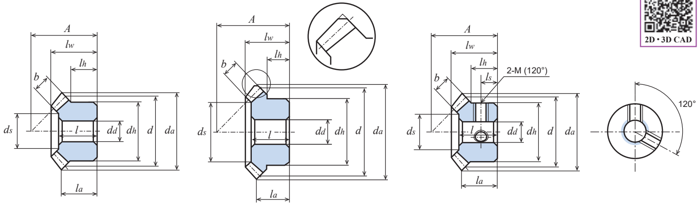
Fig. 1 (Tip chamfering)
