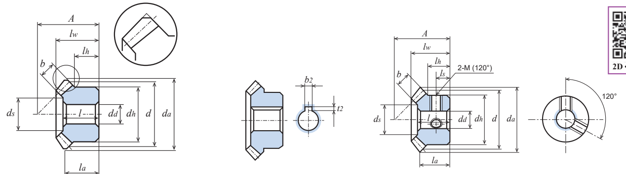
图1 (齿顶部倒角略图)
