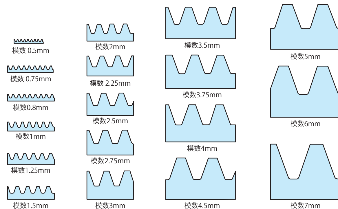
图1-1 模数的大小
