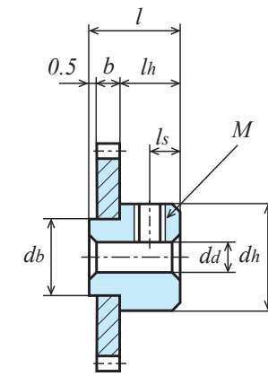
B2形状 (铆接轮毂)
