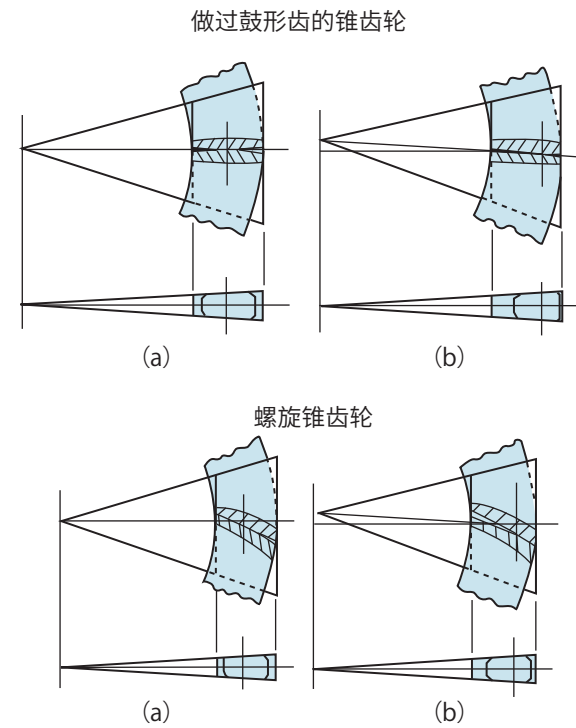
两个图均为(a)为正常位置的安装,(b)为小齿轮的圆锥顶点位置错位时的安装。请注意观察齿印位置的变化。
